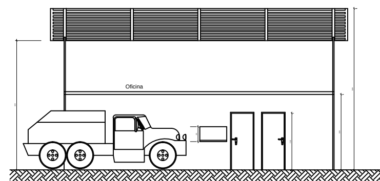
CORTE.A-A
