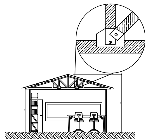
CORTE.A-A
