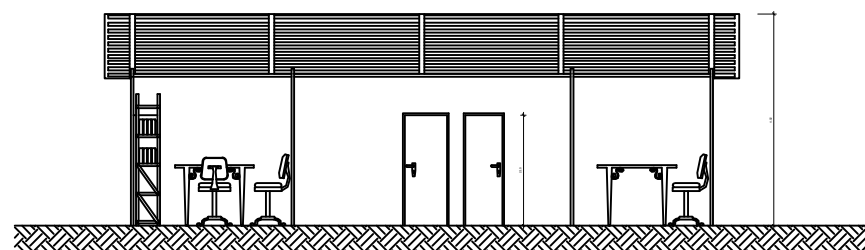
CORTE.A-A
